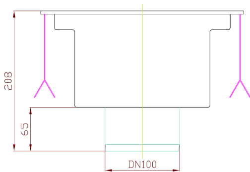
Front aanzicht
